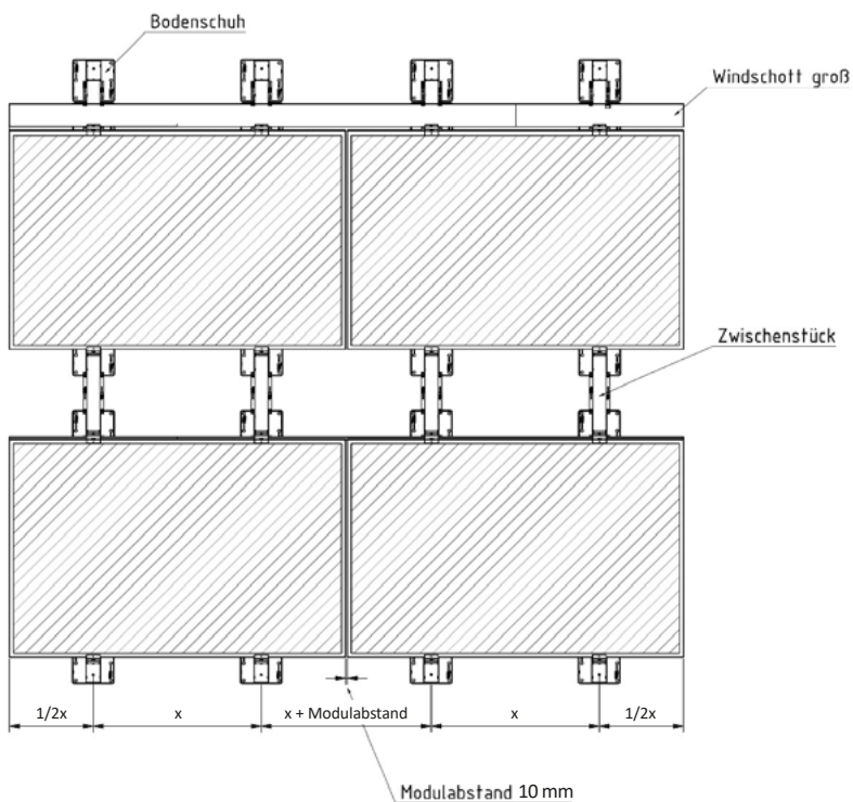
Abb.: 12.2b Aufmaß SL Fast Flat SÜD-System Viertelpunktclammung
